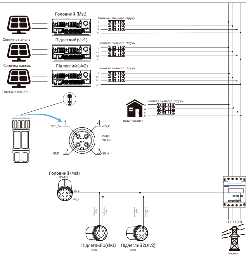
Рис. 7.29 Схема підключення Eastron (таблиця пропускну́ї здатності)
