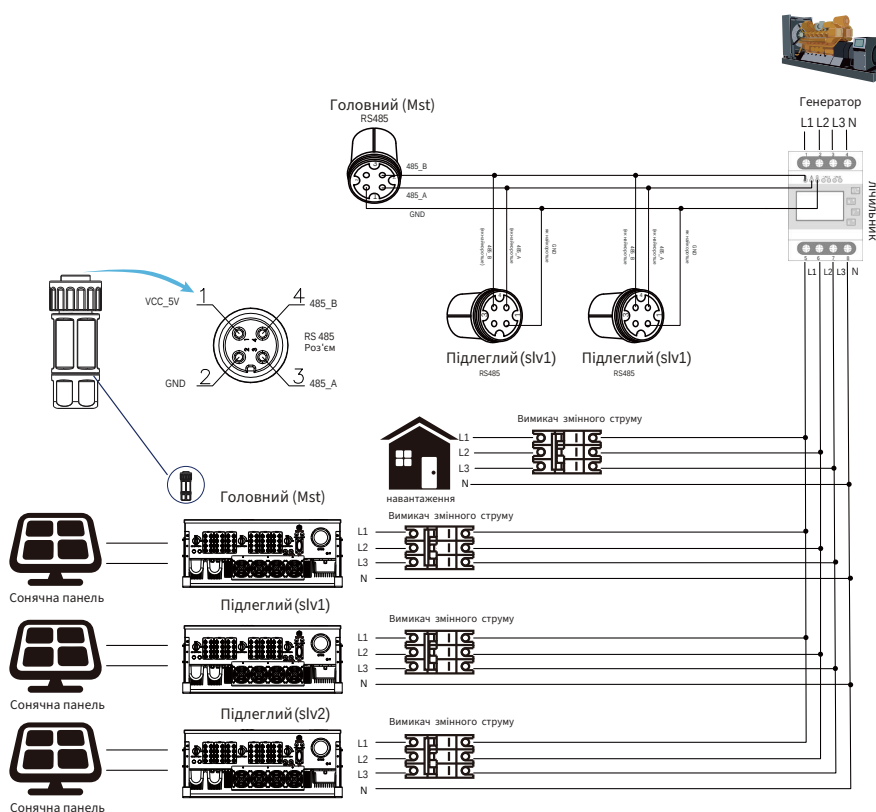
Рис. 7.23 Схема підключення Eastron (таблиця пропускної здатності)
