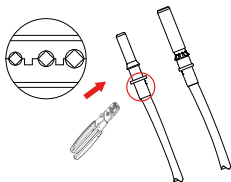
Рис. 5.4 Притисніть контактний штифт до дроту
