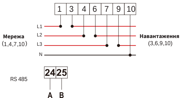
Рис. 7.11 Лічильник CHINT
