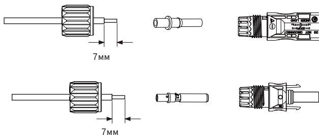
Рис. 5.3 Розбирання накидної гайки роз'єму
