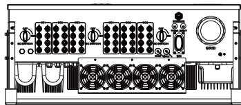
Рис. 1.2 Вид знизу
