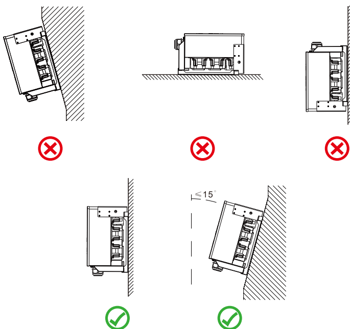
Рис. 4.2 Кут встановлення
