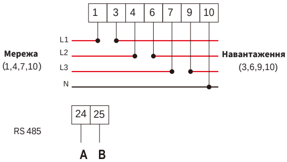
Рис. 7.30 Лічильник CHINT
