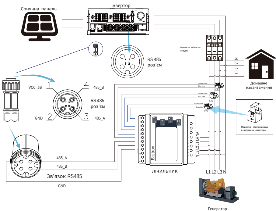
Рис. 7.8 Схема підключення лічильника Eastron
