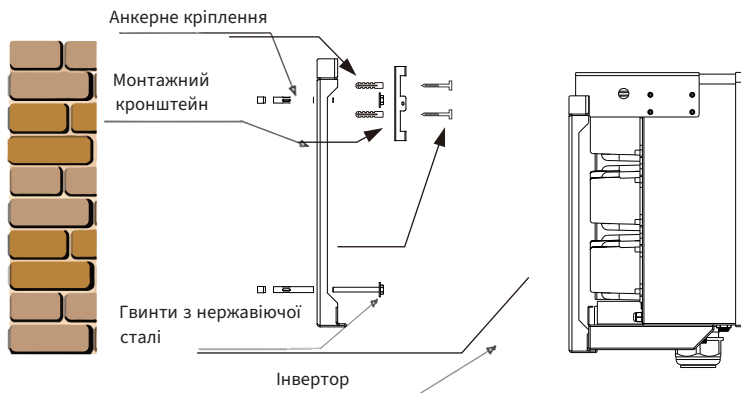
Рис. 4.5 Встановлення інвертора
