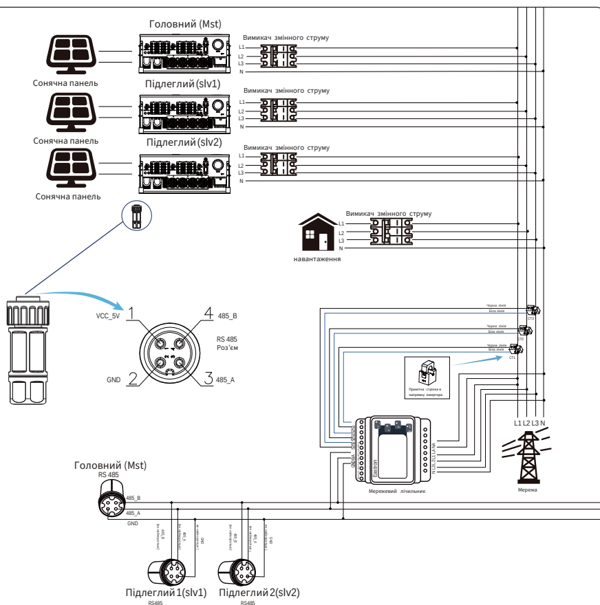
Рис. 7.25 Схема підключення (Трифазний електричний)
