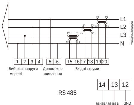
Рис. 7.5 Лічильник Eastron
