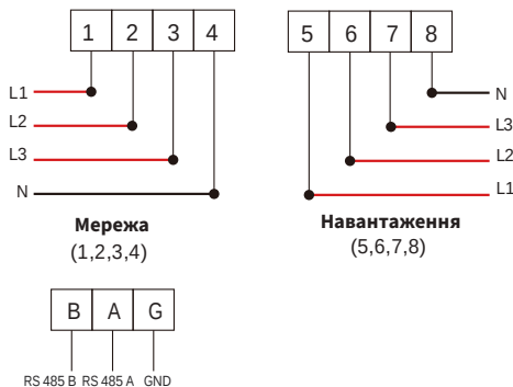
Рис. 7.3 Лічильник Eastron
