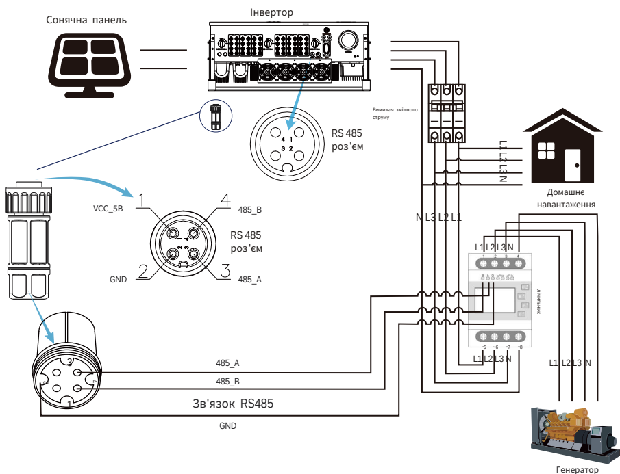
Рис. 7.4 Схеми підключення лічильника Eastron
