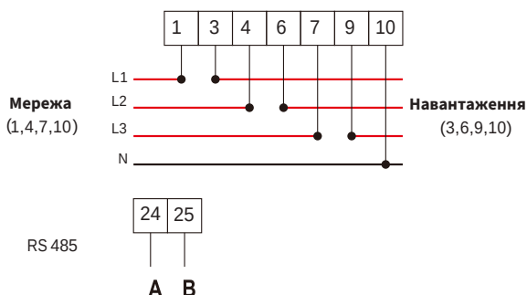
Рис. 7.28 Лічильник CHINT
