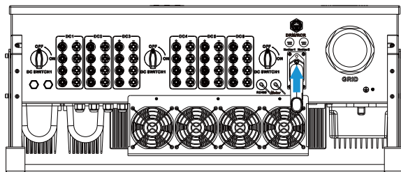
Рис. 5.14 Схема встановлення даталогера
