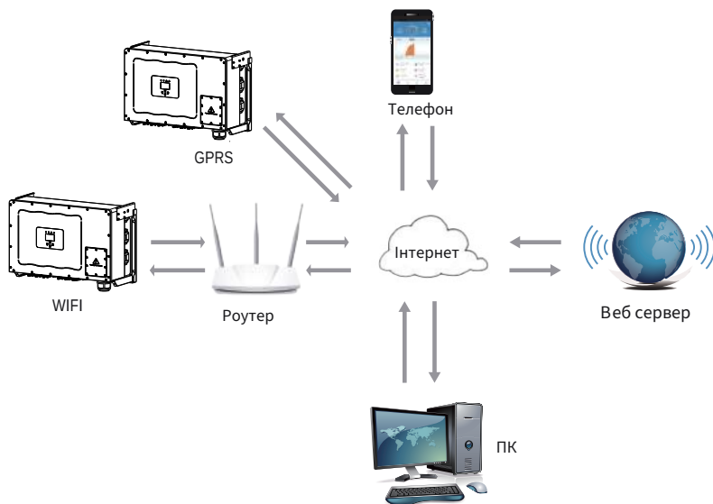
Рис. 5.13 Рішення для моніторингу через Інтернет
