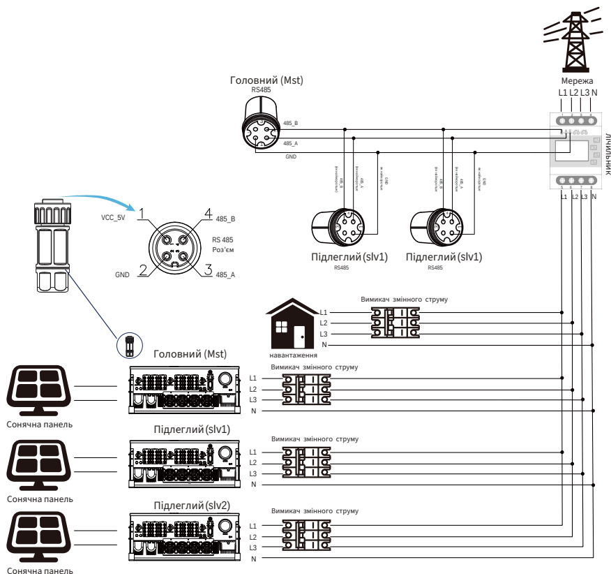
Рис. 7.21 Схема підключення Eastron (таблиця пропускну́ї здатності)
