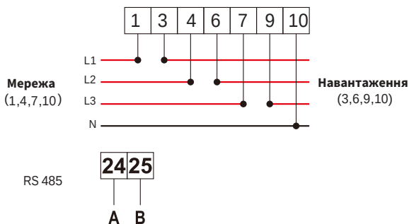
Рис. 7.9 Лічильник CHINT
