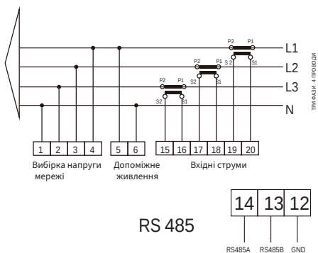
Рис. 7.24 Лічильник Eastron
