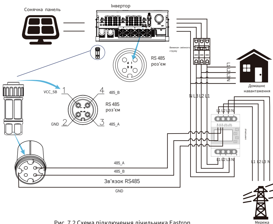
Рис. 7.2 Схеми підключення лічильника Eastron
